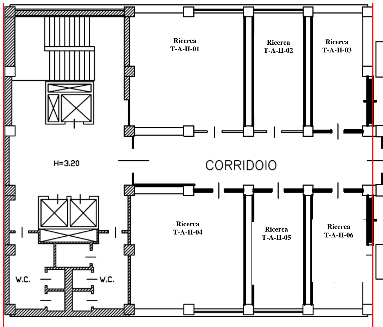
TAVOLA XIV - Studi – Edificio Triennio - PIANO II – Corpo A
